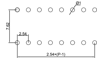
PCB开孔
